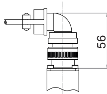
90° type Tipo 90°
